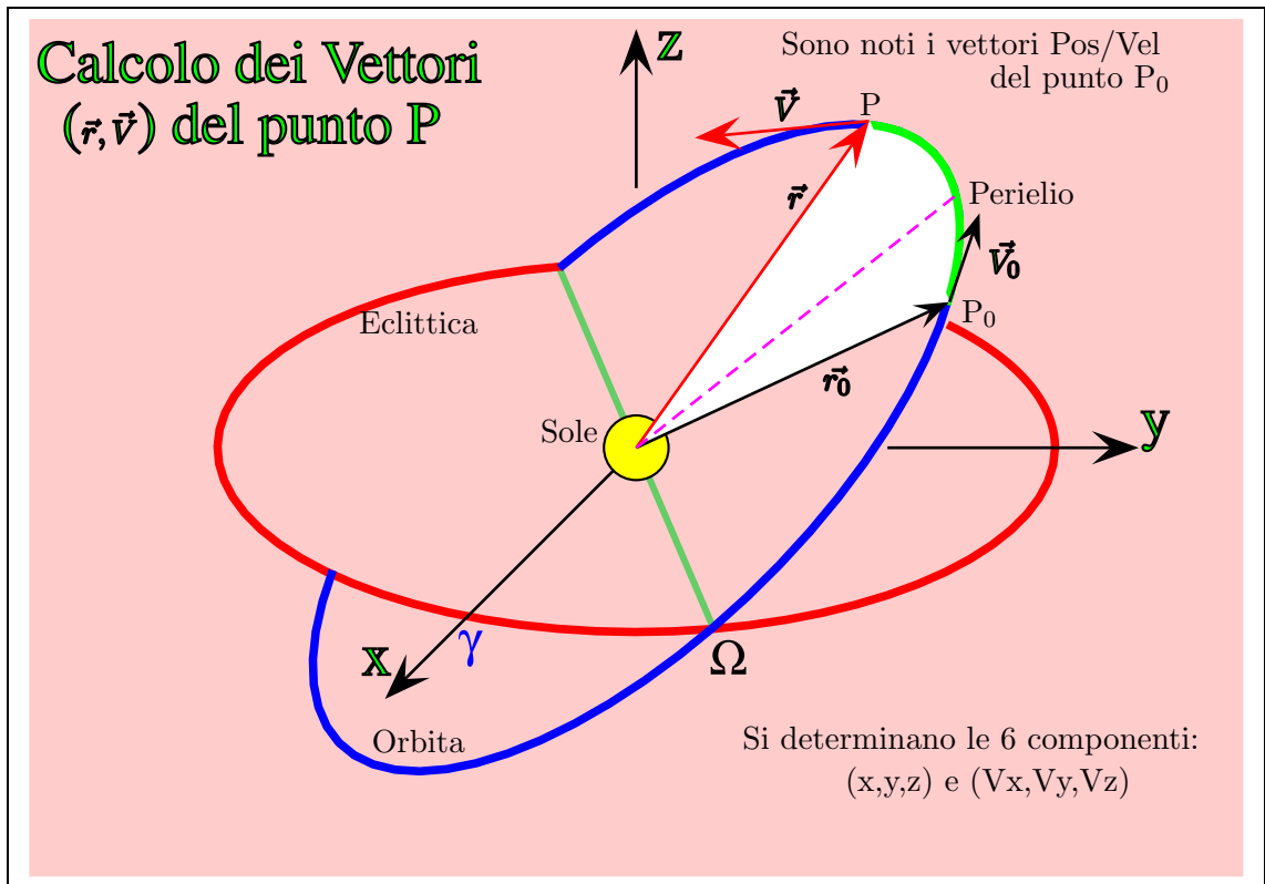
Figura 1: Vettori nello Spazio (sistema eclittico eliocentrico)
